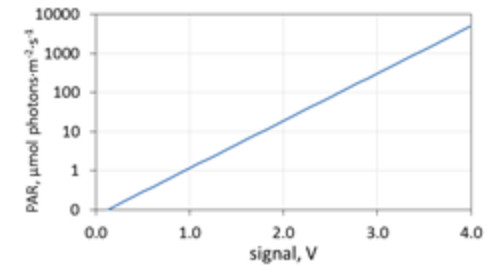
Figure 4 Logarithmic PAR Signal
